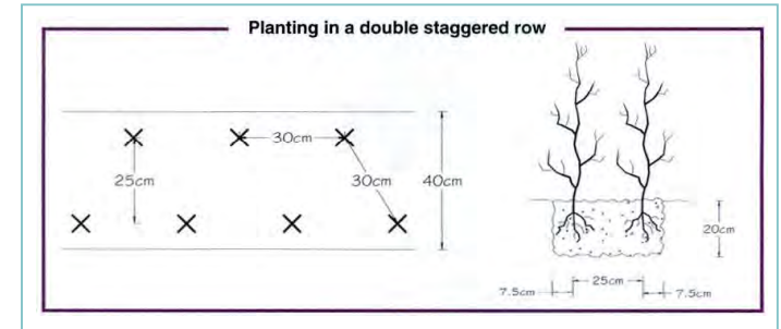
Fig N.18 Planting in a double staggered row.
